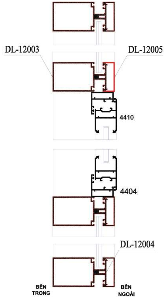
MẶT CẮT 1-1
