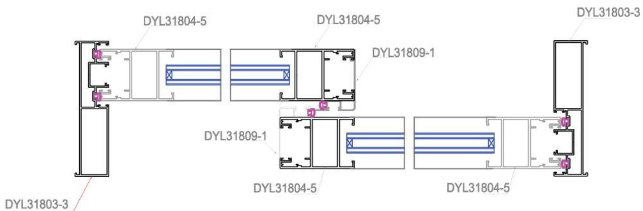
MẶT CẮT 2-2
