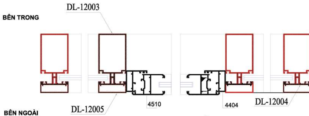
MẶT CẮT 2-2
