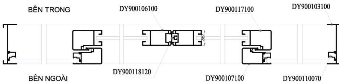
MẶT CẮT 2-2
