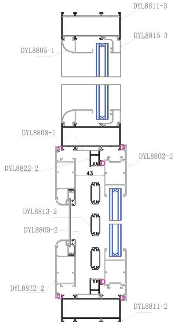
MẶT CẮT 1-2-3
