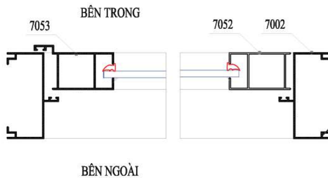
MẶT CẮT 1-1
