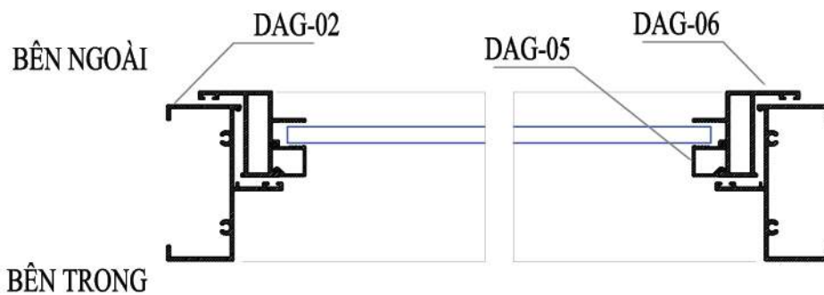
MẶT CẮT 2-2
