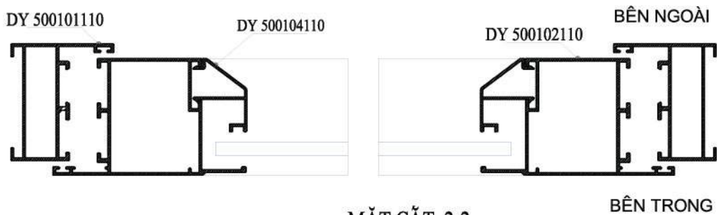
MẶT CẮT 2-2
