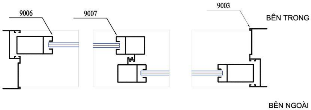
MẶT CẮT 2-2
