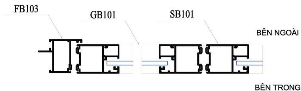
MẶT CẮT 2-2
