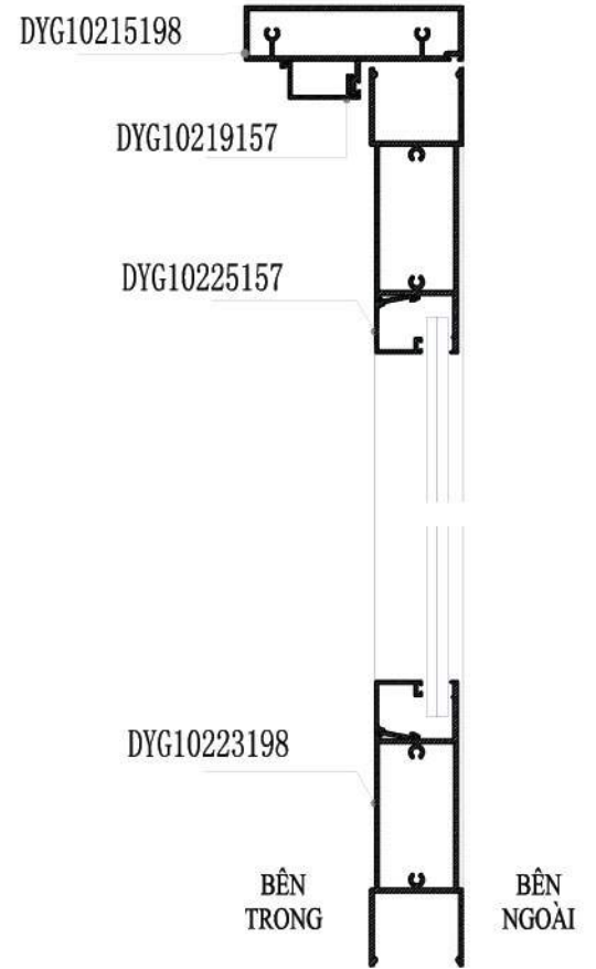
MẶT CẮT 1-1
