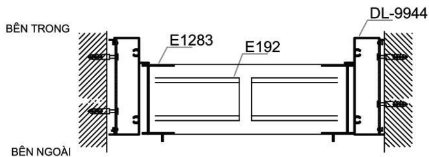
MẶT CẮT 2-2
