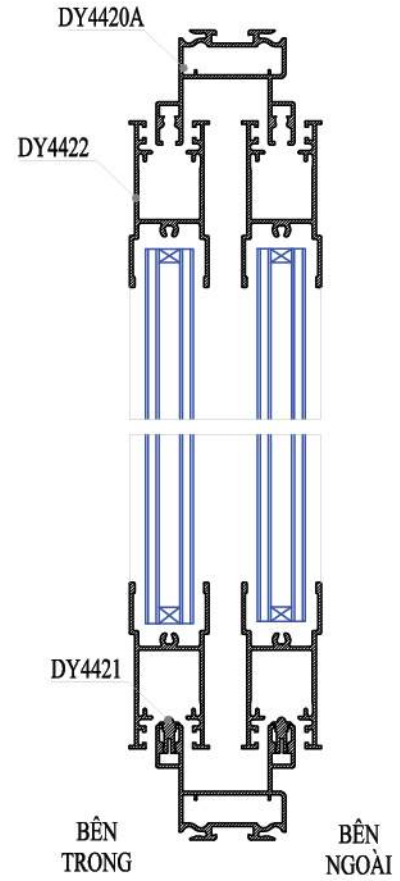
MẶT CẮT 1-1
