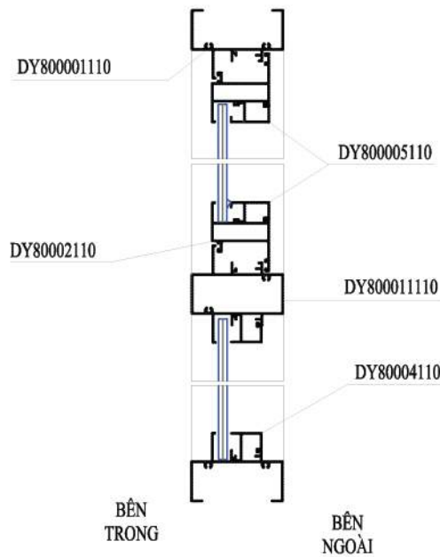
MẶT CẮT 1-1
