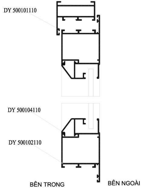
MẶT CẮT 1-1
