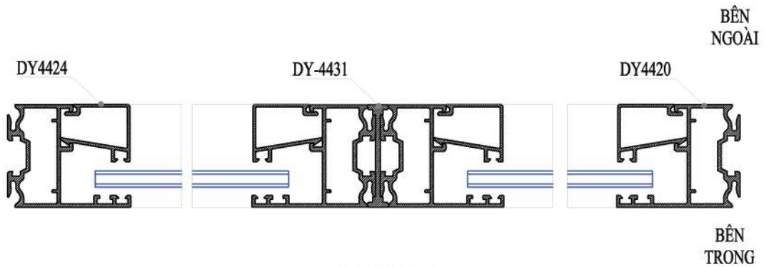
MẶT CẮT 2-2
