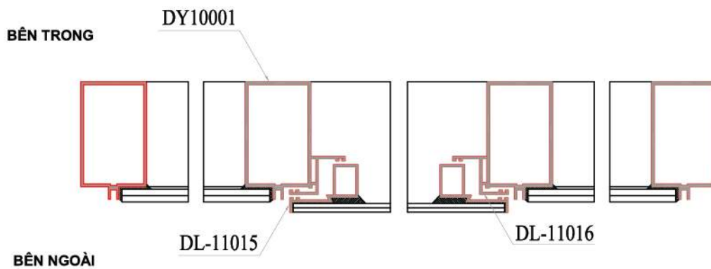
MẶT CẮT 2-2
