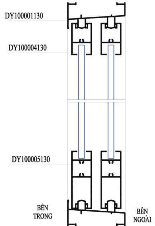
MẶT CẮT 1-1
