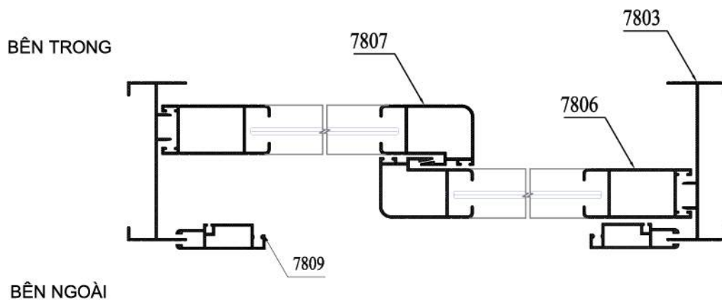
MẶT CẮT 2-2
