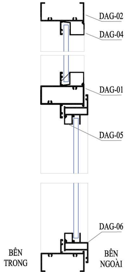
MẶT CẮT 1-1
