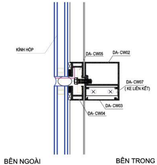
MẶT CẮT 1-1
