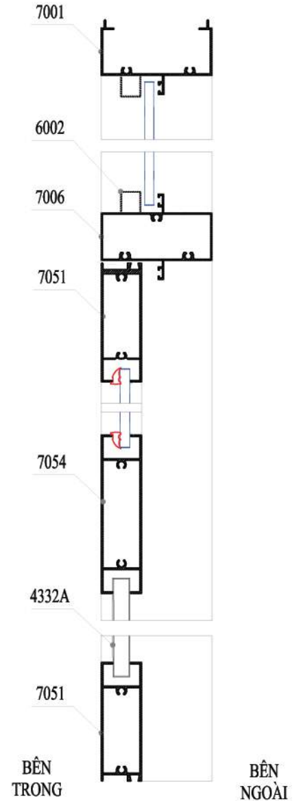
MẶT CẮT 3-3
