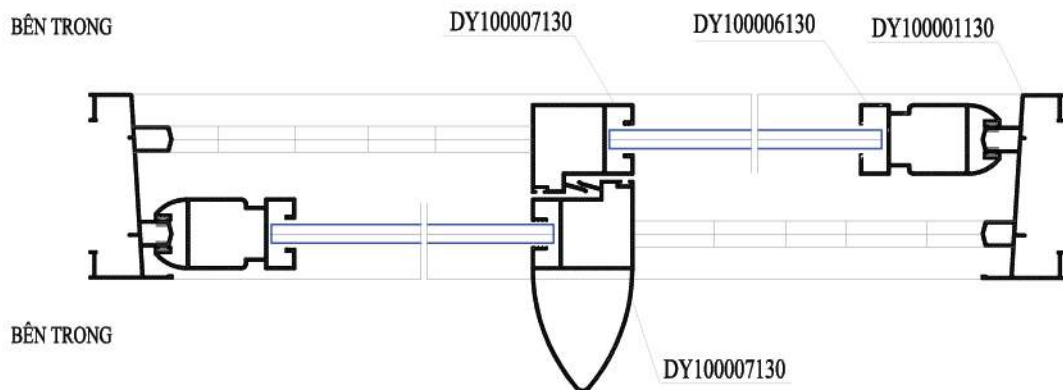
MẶT CẮT 2-2
