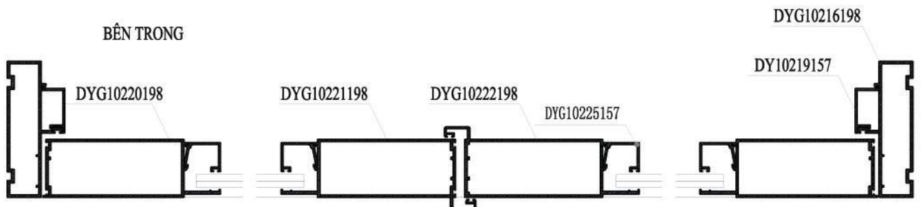
MẶT CẮT 2-2
