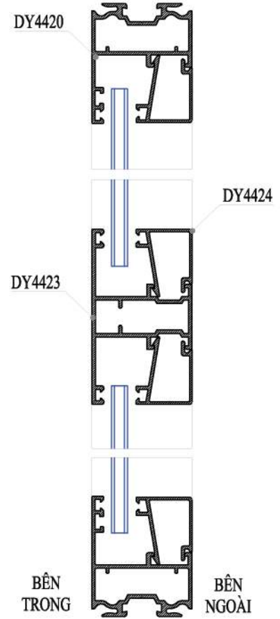
MẶT CẮT 1-1
