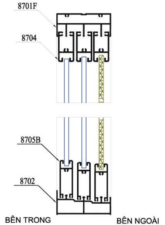
MẶT CẮT 1-1
