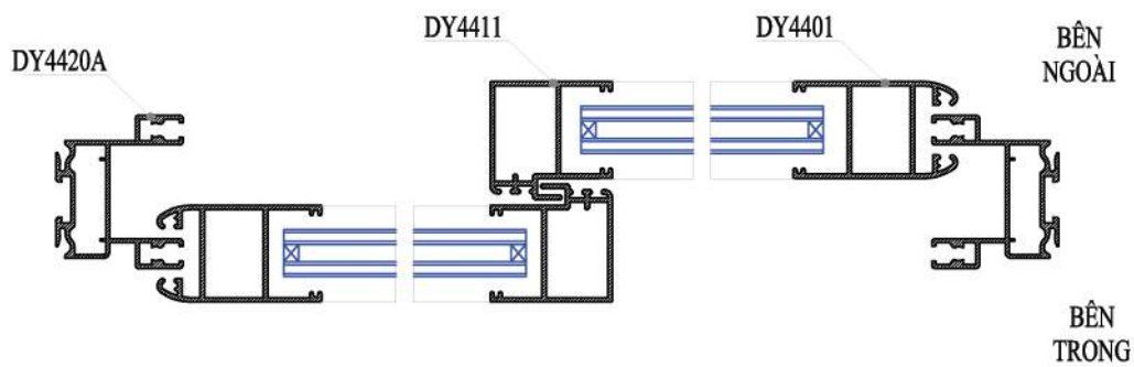
MẶT CẮT 2-2
