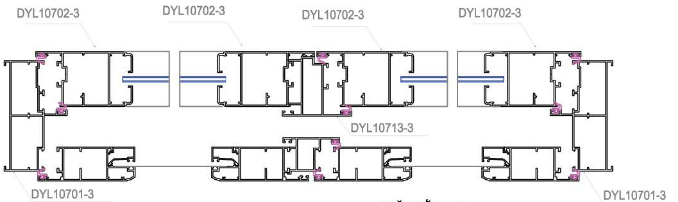
MẶT CẮT 2-2
