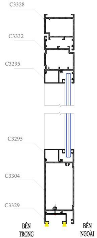
MẶT CẮT 1-1
