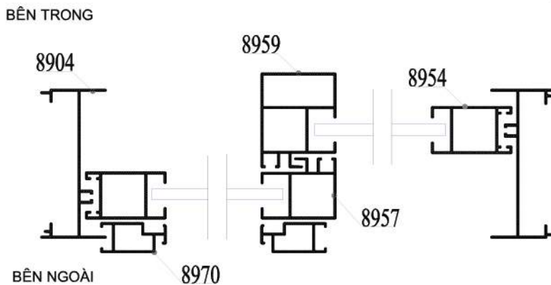
MẶT CẮT 2-2
