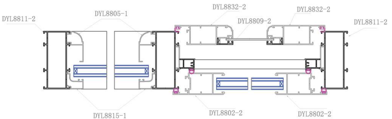
MẶT CẮT 4-5-6
