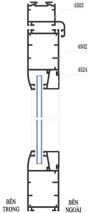
MẶT CẮT 1-1
