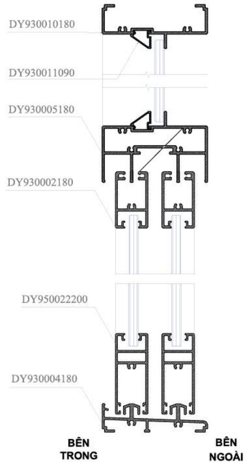
MẶT CẮT 1-1
