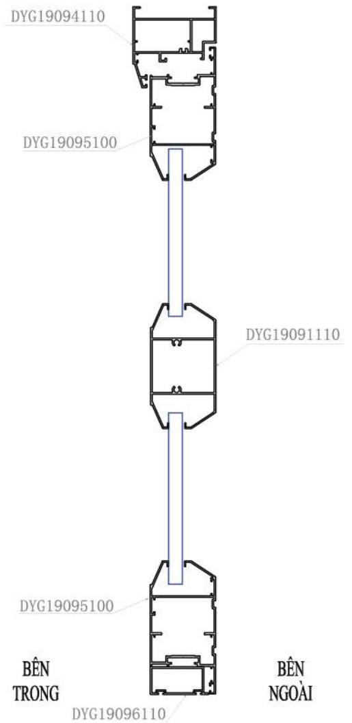
MẶT CẮT 1-1
