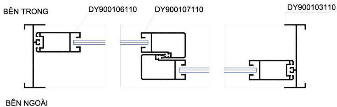
MẶT CẮT 2-2
