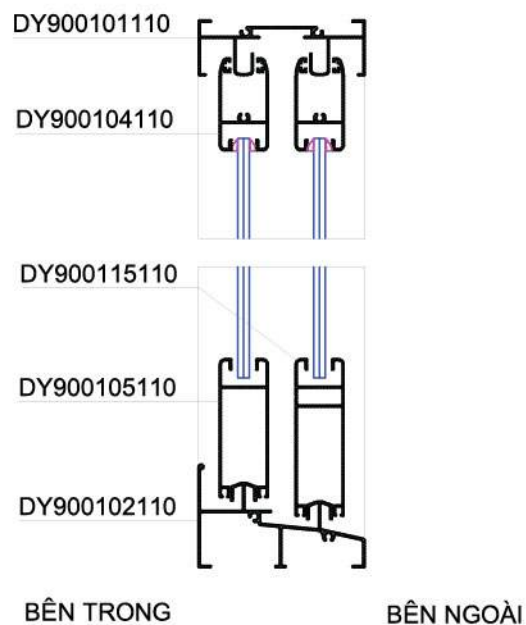
MẶT CẮT 1-1
