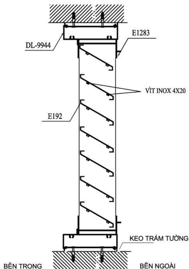
MẶT CẮT 1-1
