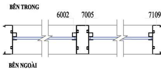
MẶT CẮT 3-3
