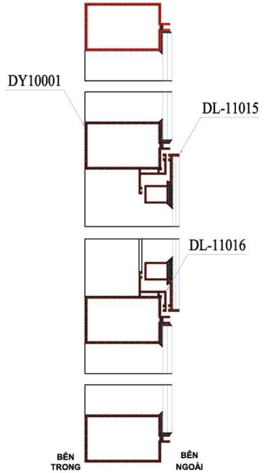
MẶT CẮT 1-1
