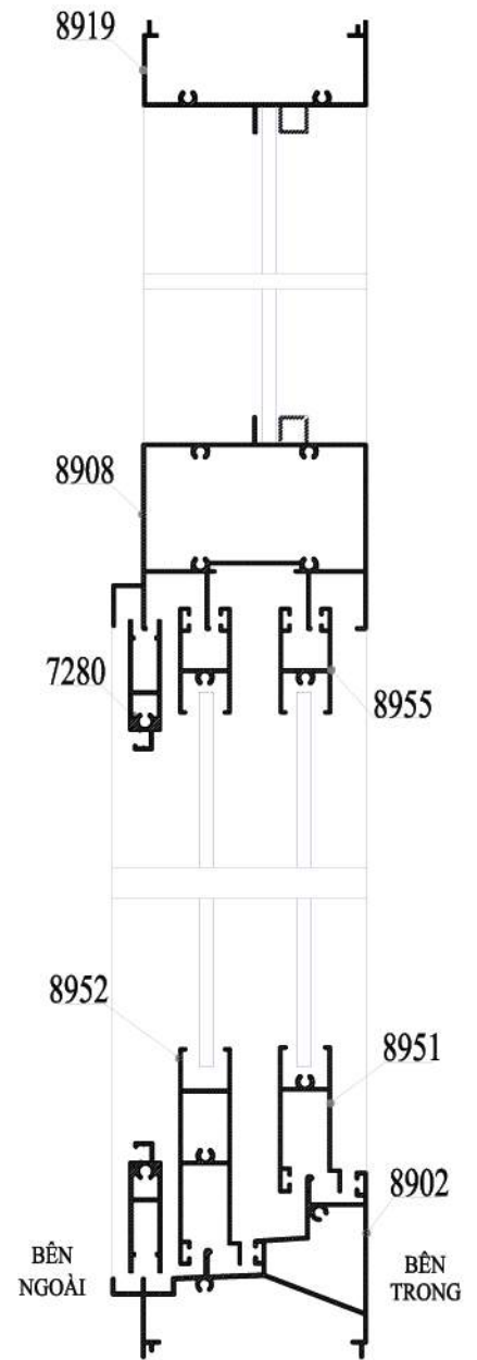
MẶT CẮT 1-1
